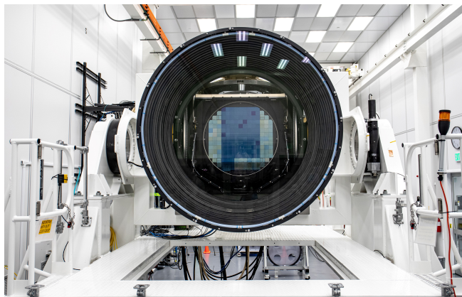
Figur 3. LSST-kameraet med dets 1,5 m brede indgangslinse og det 65 cm brede fokusplan. Foto: Jacqueline Ramseyer Orrell/SLAC National Accelerator Laboratory.
