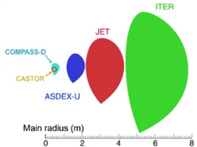
Figur 5. Tværsnit af plasmavoluminet og dets afstand fra centrum for udvalgte tokamakker og ITER. Tværsnittet af plasmaet er typisk ikke cirkulært, men snarere D-formet. Fra [5].
