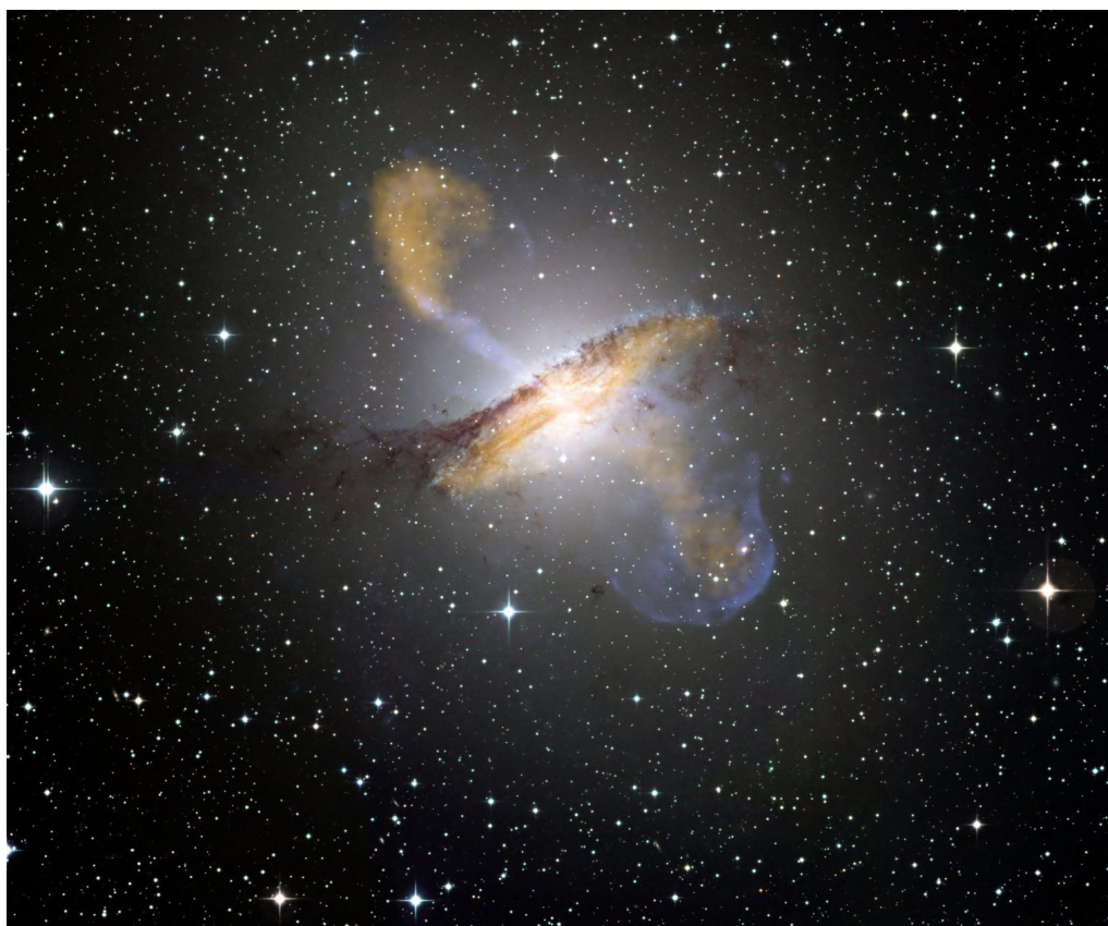
Centaurus A ligger i stjernebilledet Kentauren (Centaurus). Billedet bygger på observationsdata fra ESOs Atacama Pathfinder Experiment (APEX) teleskop i Chile, hvor man har kombineret synligt lys med submillimeter-stråling og røntgenstråling (ESO).
