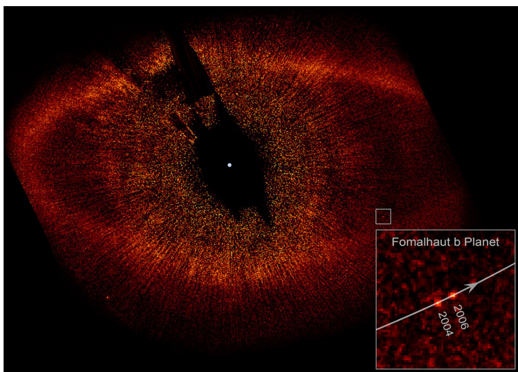
De historiske observationer fra Hubble Rumteleskopet af planeten ved stjernen Fomalhaut. Lyset fra stjernen er blændet af. Den lysende prik nederst til venstre er en baggrundsstjerne. Indsat er vist positionerne af Fomalhaut b i 2004 og 2006 (NASA/ESA).
