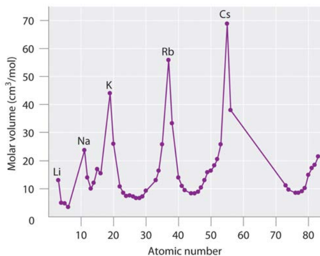
Figur 2. En moderne gengivelse af Meyers kurve, men her med atomernes rumfang plottet mod deres atomnummer og ikke deres atomvægt.
