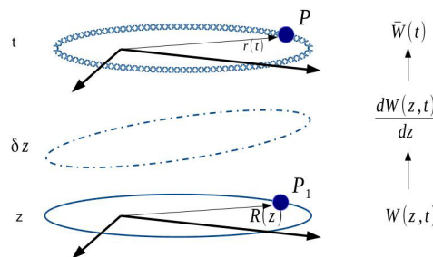
Opdelingen i den perturberede bane (øverst) i en fiktiv keplerbane (nederst) og perturbationerne (i midten). Til venstre er tidsangivelserne givet, til højre ses hvordan Hansen skifter mellem systemerne.
