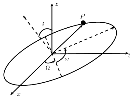
Illustration af baneelementerne. Middelanomalien M er ikke vist da den er defineret på en omskrevet cirkel således at M varierer lineært med tiden.
